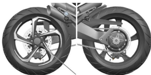
Nakrętki M12 X 1.5 Moment obrotowy dokręcenia nakrętki koła tylnego: 110N.m.
